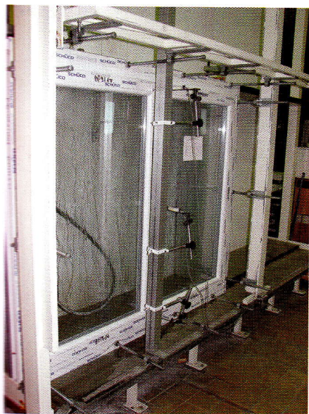
3. kép – Középen felnyíló kemény PVC-ablak a vizsgálóberendezésen
