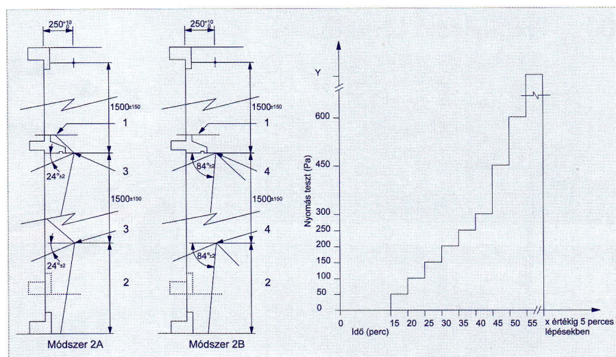
1-2. kép – A víz permetezésének módja és nyomásfokozatai vízszintes osztással rendelkező szerkezethnél a csapóesőnek kitett és védett helyszínt szimulálva
